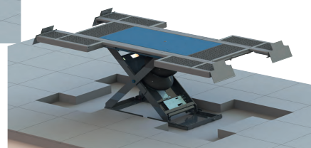
HLS3513-14 埋込仕様
